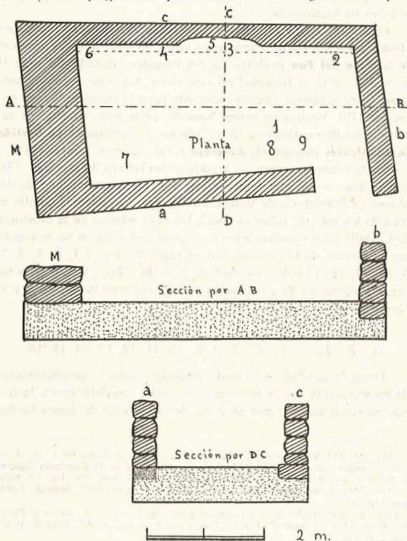
Fig. 19.—Planta y secciones de la habitación número 1 del poblado de la Torre del Mal Paso.
