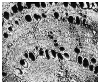
Plànol transversal del carbó prehistòric de roure menut. Plano transversal de carbón prehistórico de quejigo
