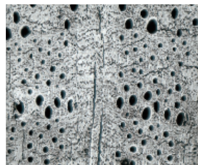
Plano transversal de carbón prehistórico de carrasca o coscoja.
