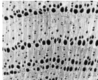
Pla transversal de carbó prehistòric de freixe. Plano transversal de carbón prehistórico de fresno
